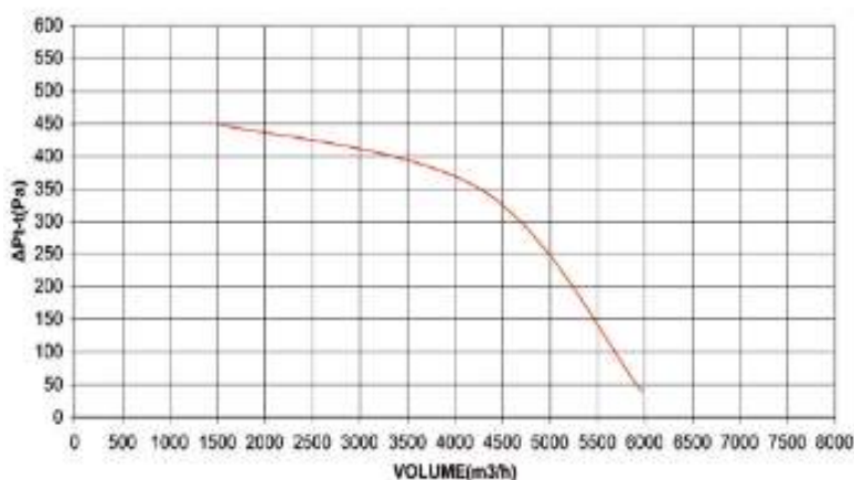
Ø250-1.5HP-1450RPM
